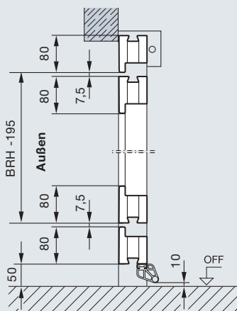
Kiptor ET 500 mit Schlupftür
