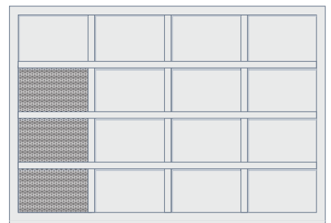
Motiv 499 , Beispiel mit Aluminiumblech- und asymmetrisch angeordneter Streckgitter-Füllung
