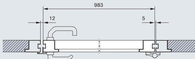
Kiptor ET 500 mit Schlupftür
